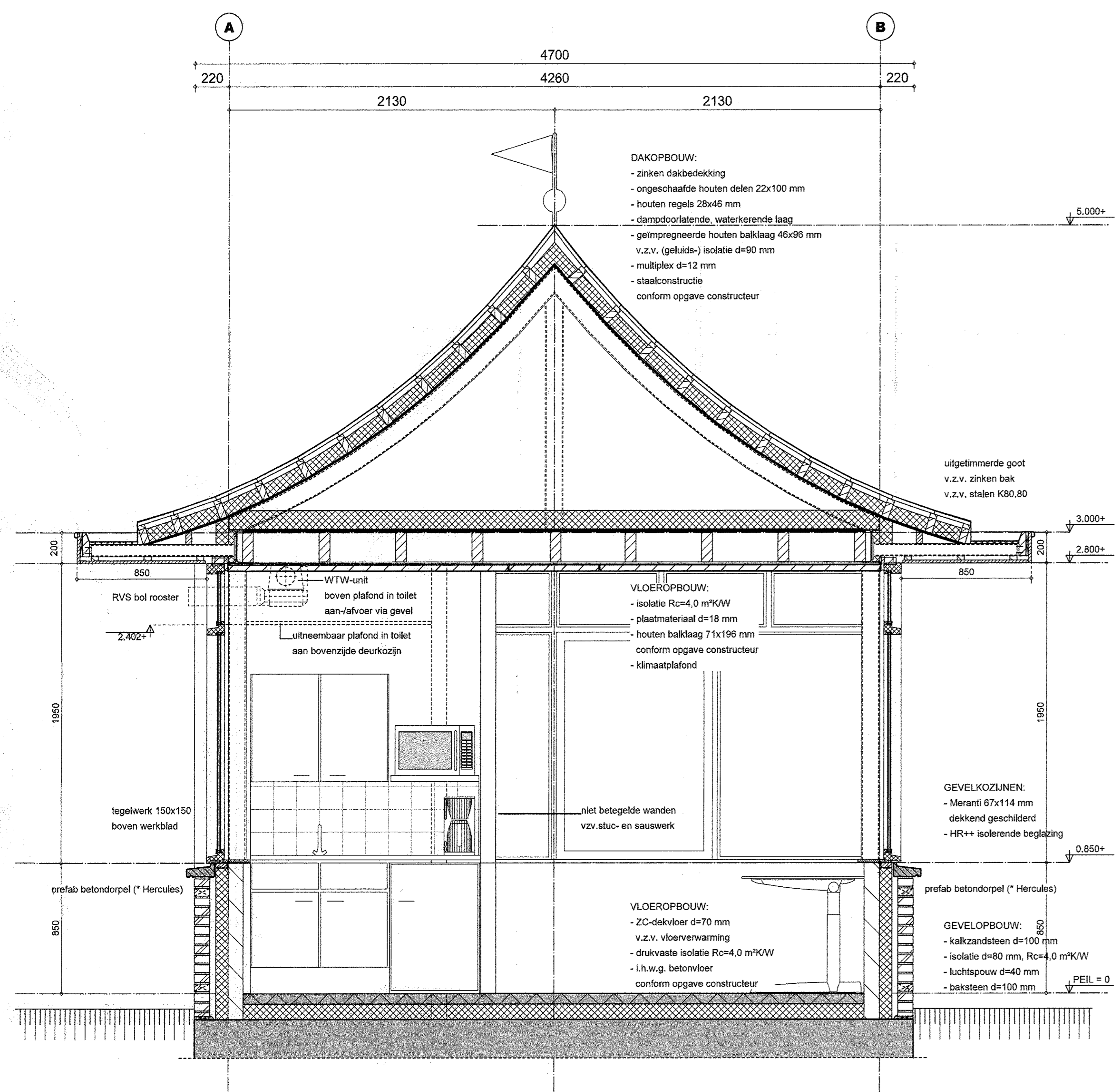
DOORSNEDE - schaal 1:20 -
